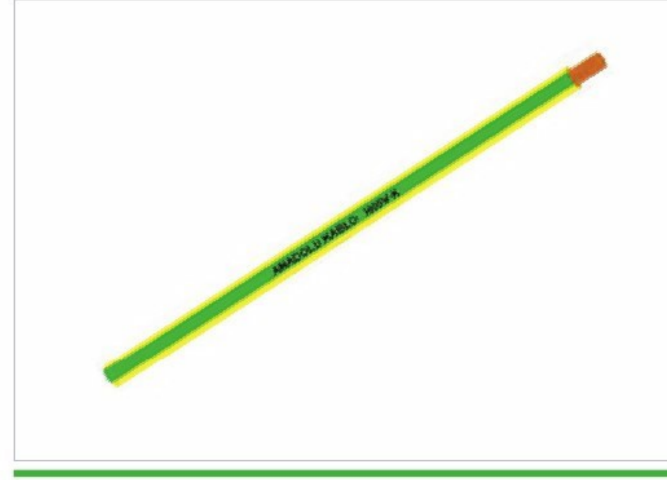
H05V-K (NYAF) 300/500 V
